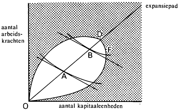
Figuur 3. Isoquantendiagram
