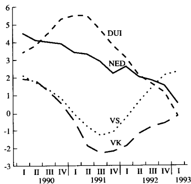
Figuur 4. Volumegroei bruto binnenlands produkt, proc. jaarmutaties van voortschrijdend 4-kwartaalsgemiddelde
