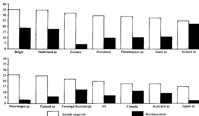
Figuur 1. Sociale uitgaven (in procenten van het bbp, 1981) en werkloosheidspercentage (derde kwartaal 1984)
